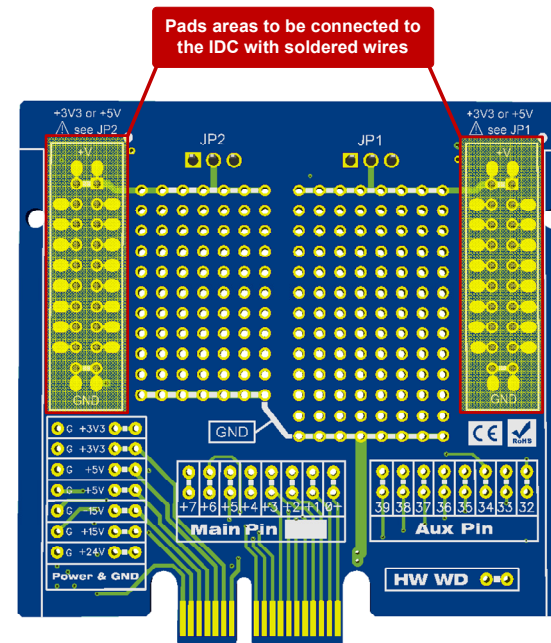
Bottom side
